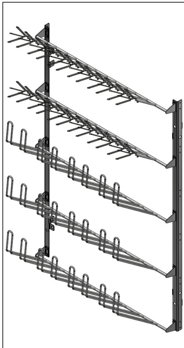
Vægskinnesæt til 5 rækker
